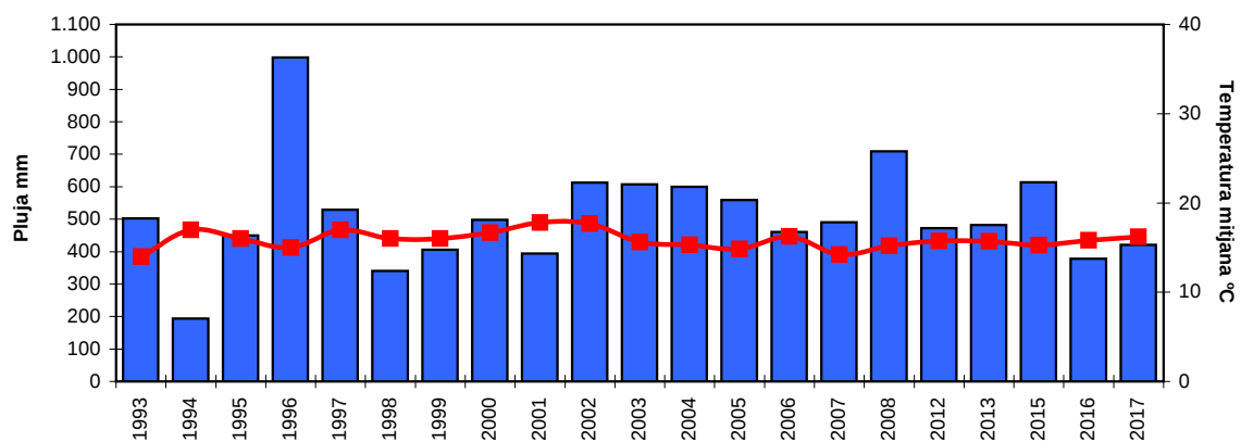
Evolució de la temperatura i la pluviometria de Terrassa 1993-2008, 2012-13 i 2015-2017
