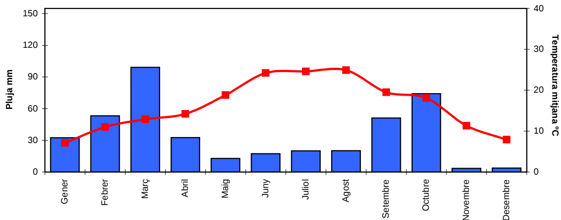
Evolució anual de la temperatura i la pluviometria de Terrassa 2017
